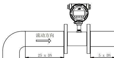
在同一个平面上 一个90度弯头
