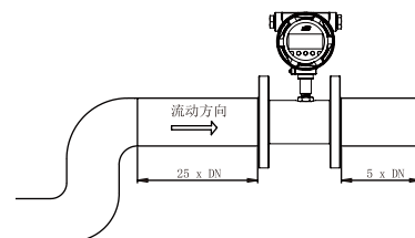
在同一个平面上 两个90度弯头
