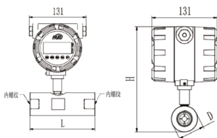
尺寸图2 (内螺纹连接型)
