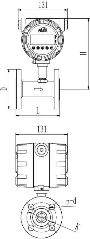
尺寸图3 (PN16法兰连接型)
