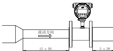
缩管
