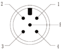
M12接插件
