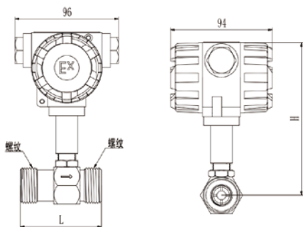
尺寸图2 (螺纹连接型)
