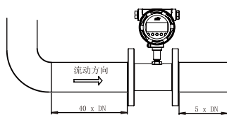
在不同一个平面 上一个90度弯头
