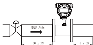
全开阀门
